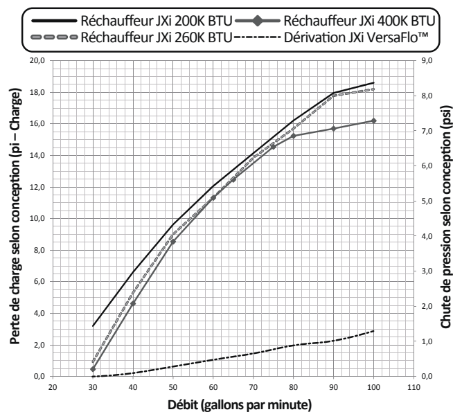
Figure 1. Graphique de perte de charge
